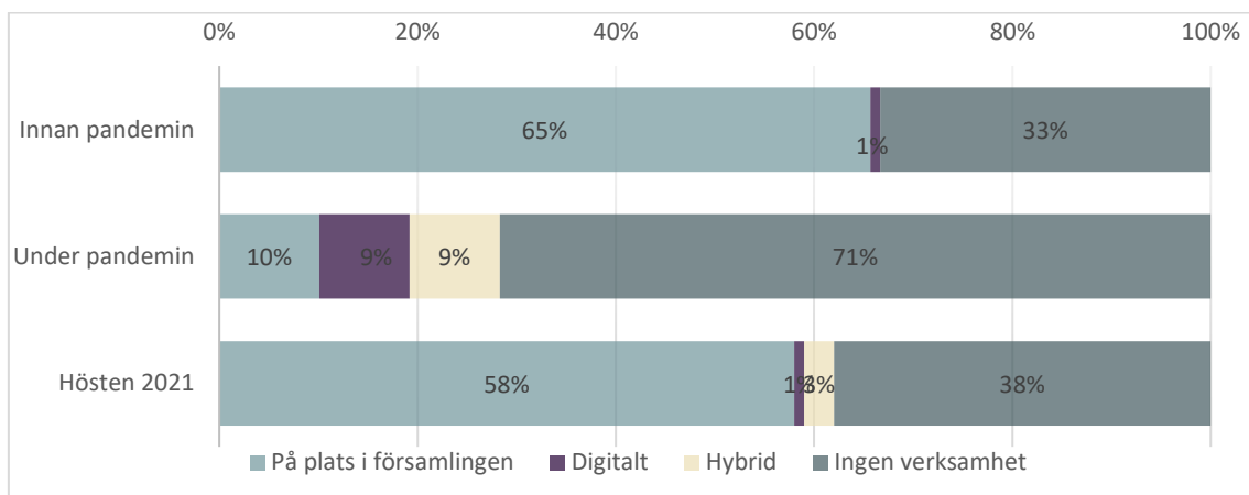
Figur 15. Musikverksamhet
